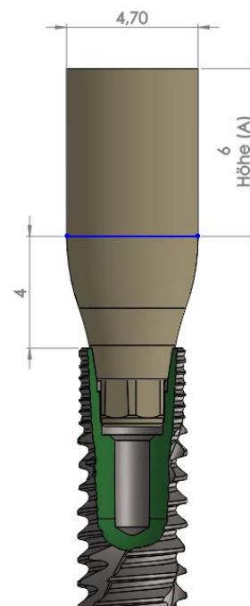
Meoplant mit Heilkappe (Maße in mm)
