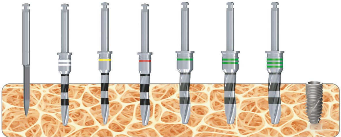
Bohrprotokoll - Implantat Ø 4,2mm - Knochenqualität: D1
