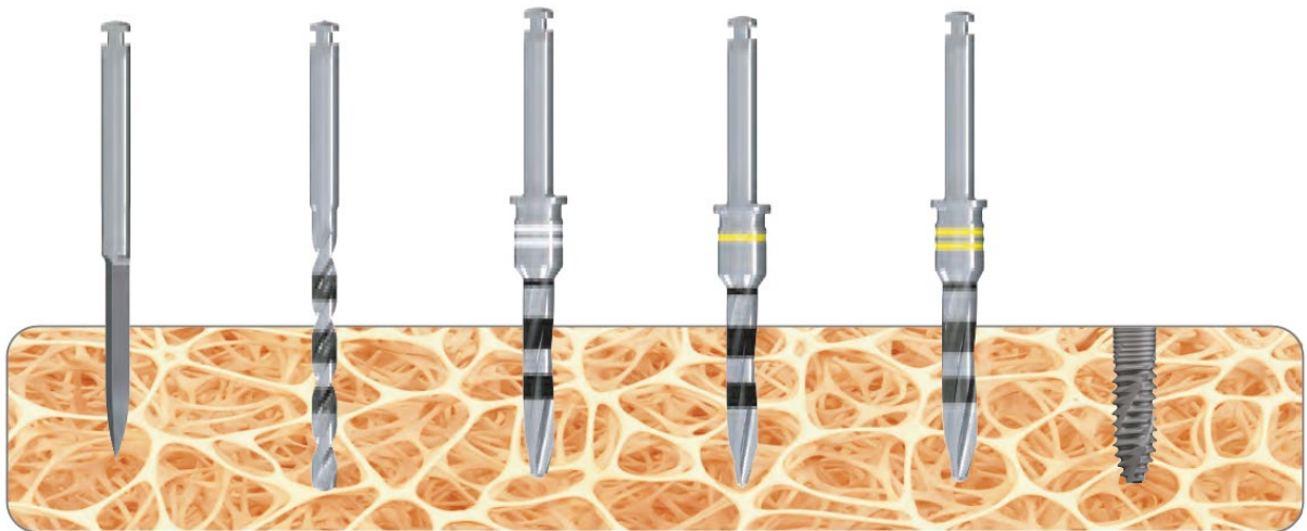
Bohrprotokoll - Implantat Ø 3,5mm - Knochenqualität: D2 – D3
