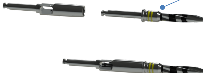
Zusammenbringen der Bohrererlängerung mit dem Parallelbohrer
