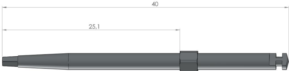
1.4 Sechskantinstrument / ISO-Schaft
