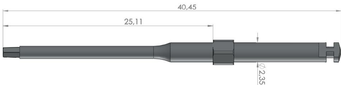
1.2 Sechskantinstrument / ISO-Schaft
