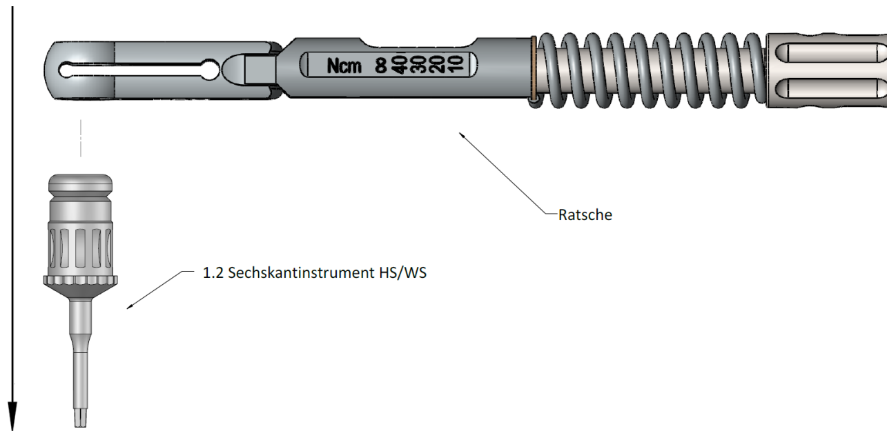
1.2 SECHSKANTINSTRUMENT HS/WS – RATSCH
