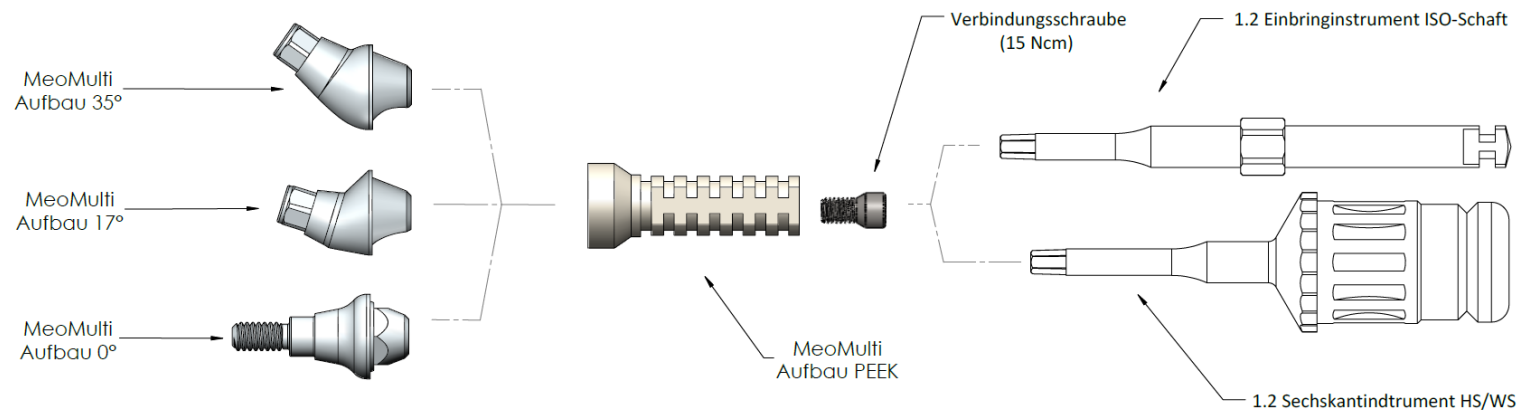
MEOMULTI AUFBAU PEEK • 1.4 SECHSKANTINSTRUMENT ISO-SCHAFT • VERBINDUNGSSCHRAUBE
