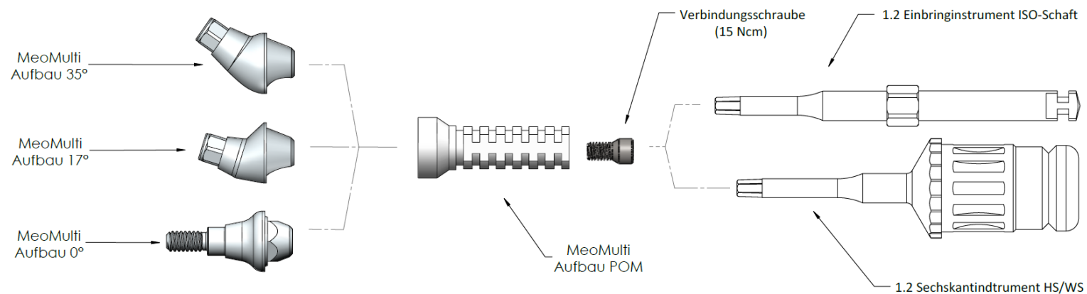
MEOMULTI AUFBAU POM • 1.4 SECHSKANTINSTRUMENT ISO-SCHAFT • VERBINDUNGSSCHRAUBE
