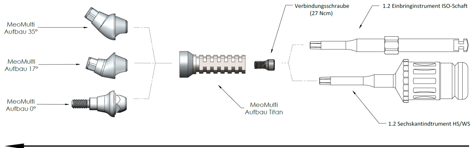
MEOMULTI AUFBAU TITAN • 1.4 SECHSKANTINSTRUMENT ISO-SCHAFT • VERBINDUNGSSCHRAUBE CAD/CAM
