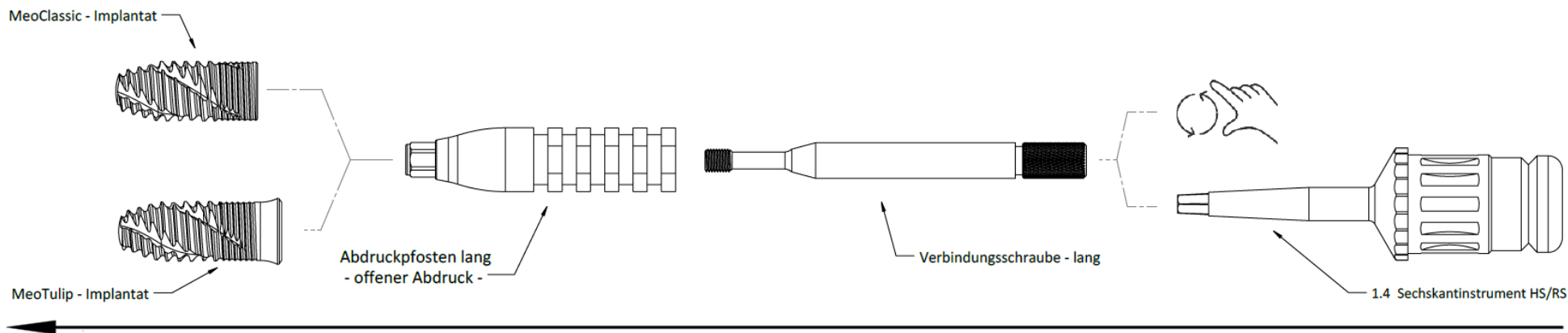
ABDRUCKPFOSTEN OFFEN - LANG – 1.4 SECHSKANTINSTRUMENT HS/RS VERBINDUNGSSCHRAUBE KURZ
